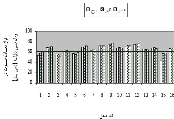
نمودار ۱: مقایسه‌ی تراز معادل شدت صوت در سه نوبت روزانه در استان زنجان با استاندارد سازمان حفاظت محیط‌زیست ایران
