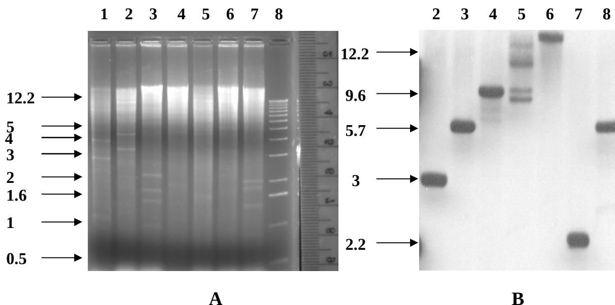
شکل 4: ساترن بلاتینگ DNA ژنومی آسپرژیلوس فومیگاتوس.
